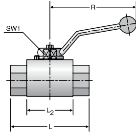
DN4-DN25
